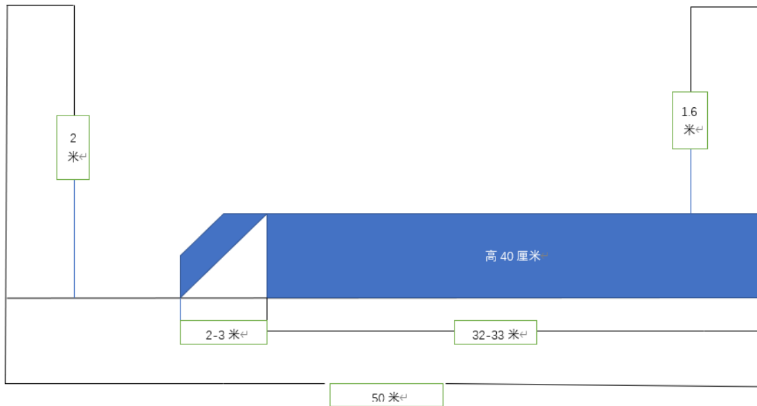
游泳馆垫层示意图
